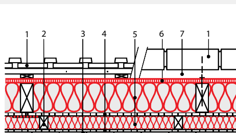
Buitenmuur lage energiewoning (houtspantenbouw)
